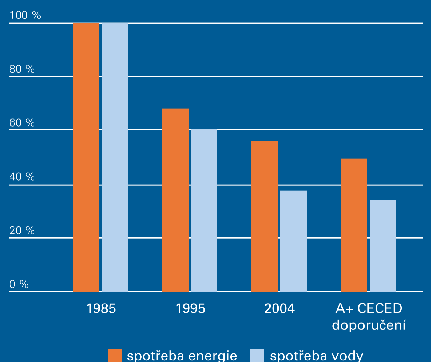
Průměrná spotřeba energie a vody automatických praček
